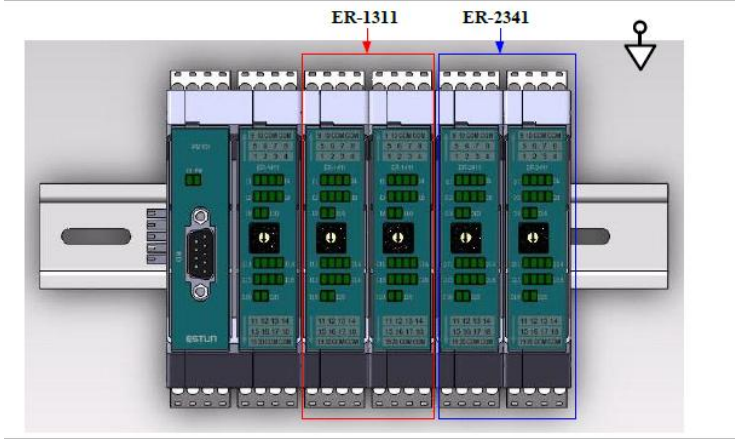
图7-13 安装顺序示例
