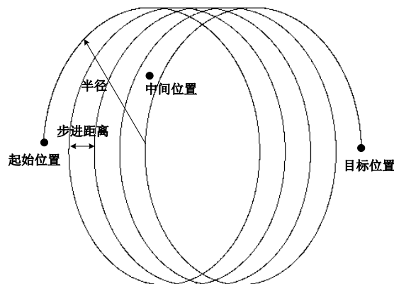
图11-17 MovH 螺旋运动关键点示意
