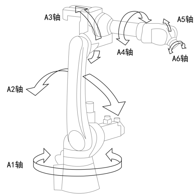
图6-1 关节坐标系下的各轴动作示意
