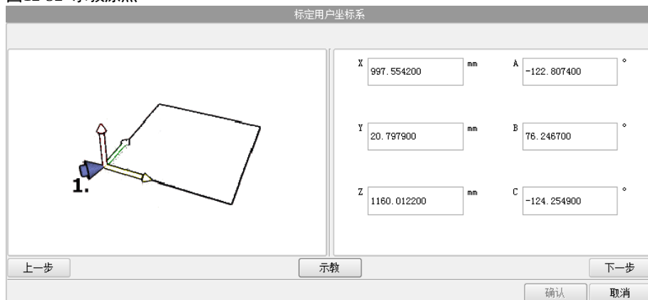
图12-52 示教原点
