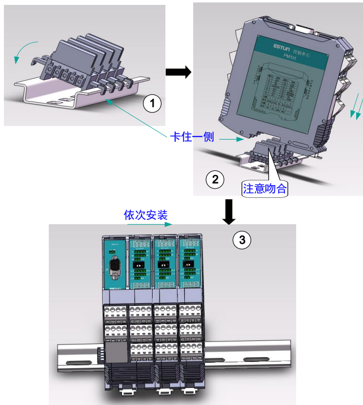
图 7-12 模块的安装示意图
