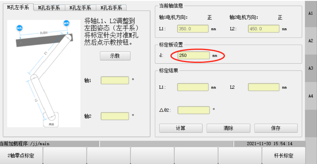
图12-109 标定板设置
