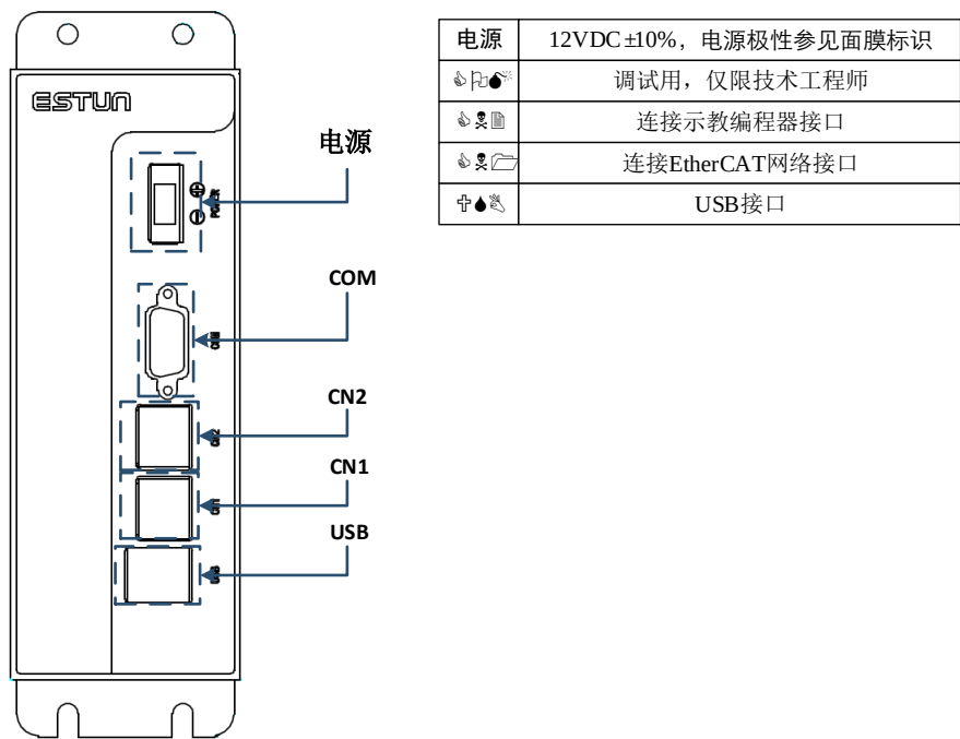
图7-5 控制单元的接口布局
