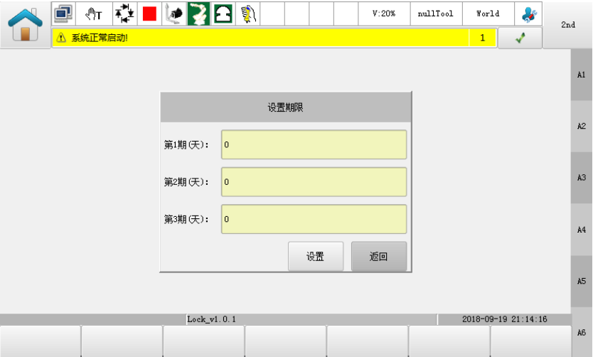
图12-68 设置期限
