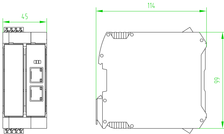
图7-19 耦合器尺寸图
