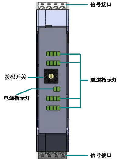
图7-10 数字输入 ER-1311 接口图示
