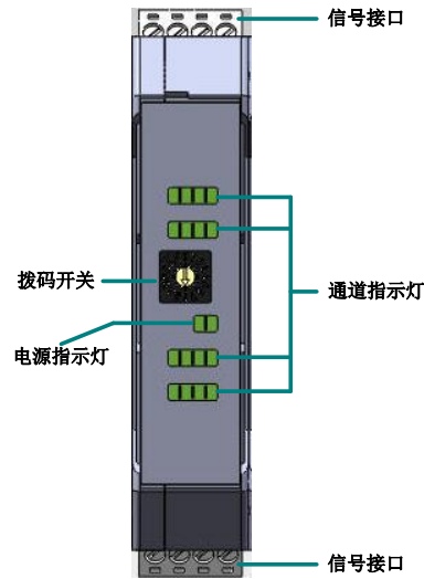
图7-11 数字输出 ER-2341 接口图示
