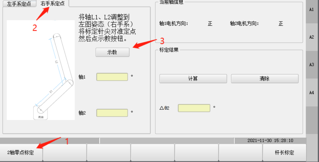
图12-103 右手系标定
