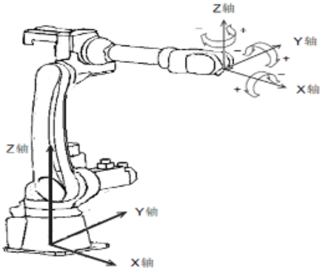
图8-2 直角坐标系下各轴的运动方向
