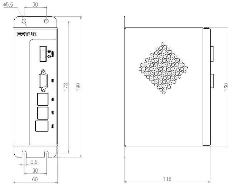
图7-6 安装尺寸图
