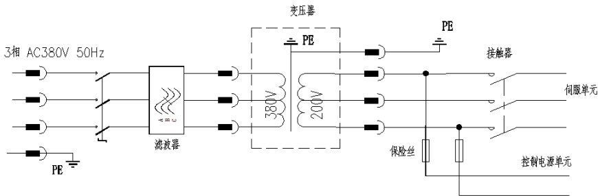
图7-4 电源的输入连接
