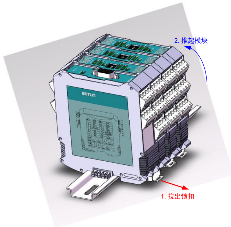
图7-15 拆卸示意图
