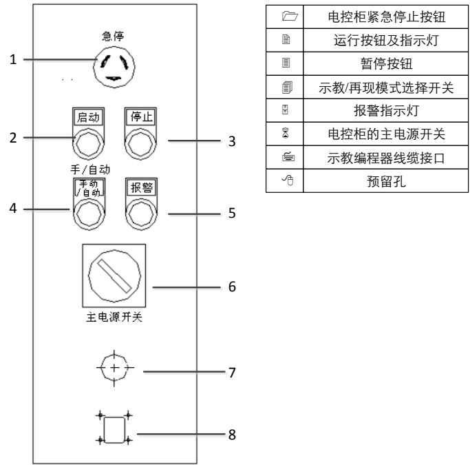
图7-2 电控柜按钮分布
