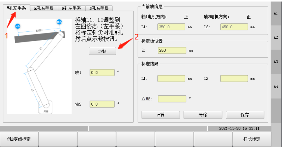
图12-105 M 孔左手系
