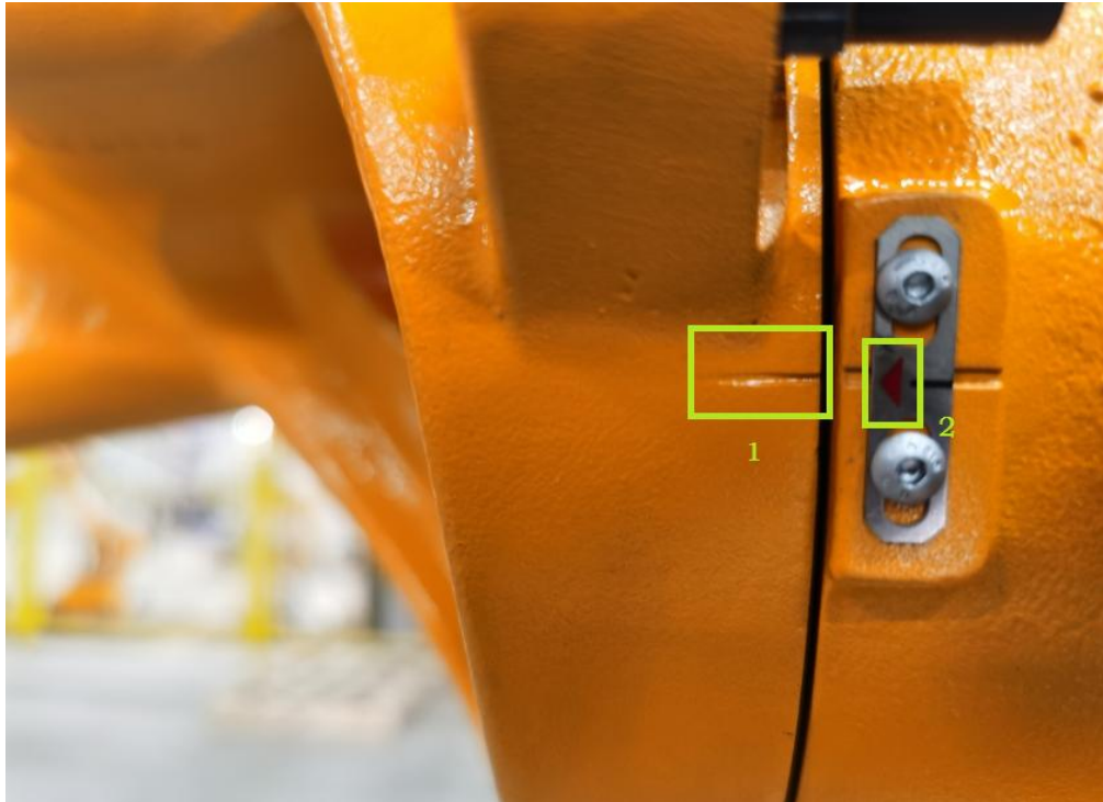
图12-89 本体上轴的零标刻度线图
