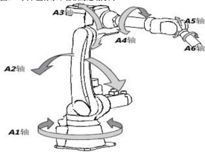
图8-1 关节坐标系下各轴的运动方向
