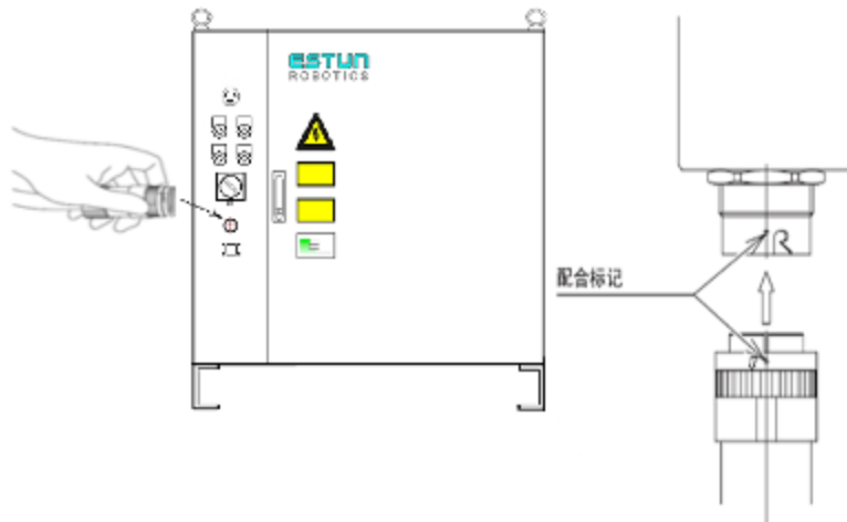
图4-3 示教编程器与电控柜的连接示意图
