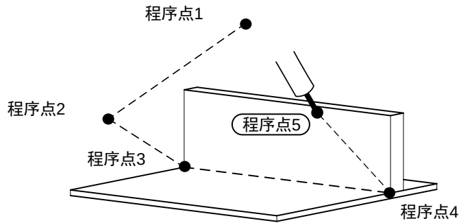
图8-13 示教程序点 5
