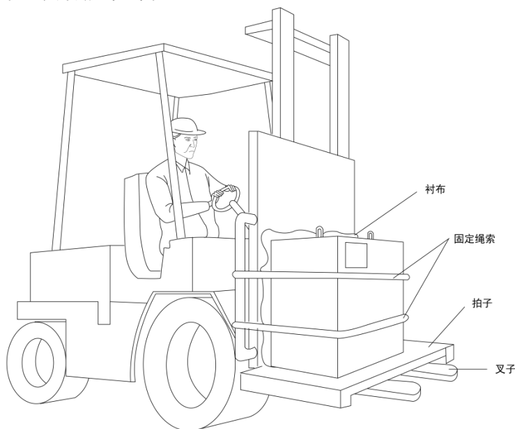
图3-1 叉车搬运示意图
