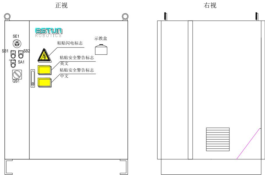
图7-1 控制器外观
