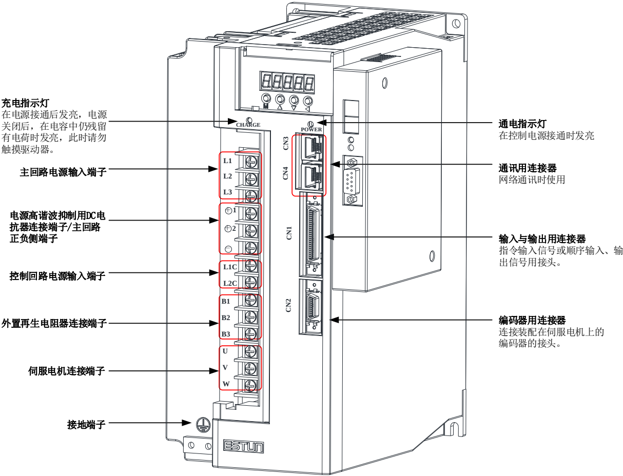
图7-8 驱动器接线端口及功能分布
