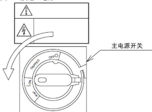
图5-1 接通主电源
