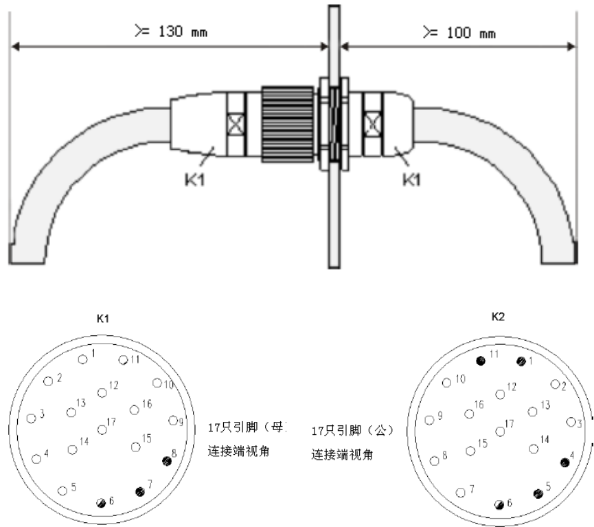
图7-26 示教编程器线缆与电控柜的连接
