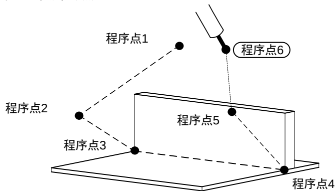
图8-14 示教程序点 6
