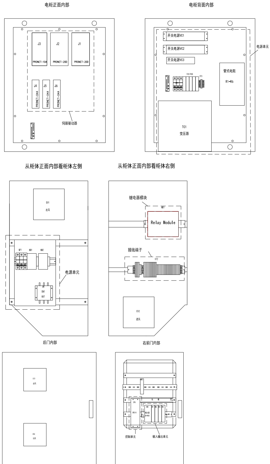
图7-3 电柜内部布局图
