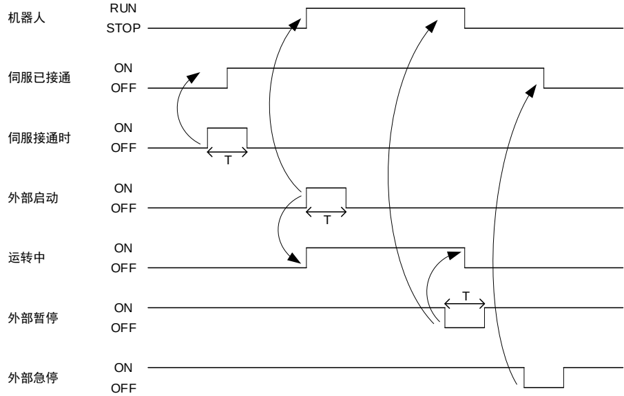
图6-2 机器人控制器启停时序图
