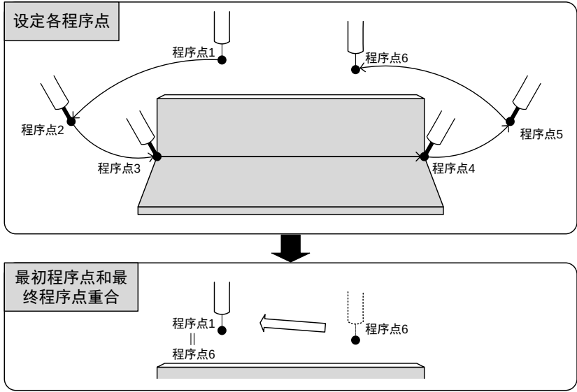
图8-7 示教程序的运行路径示意
