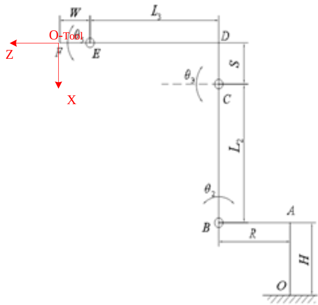
图10-1 工具&负载质量信息坐标系说明
