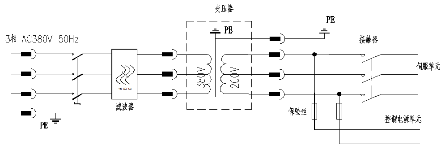
图4-2 供电电源接线示意图
