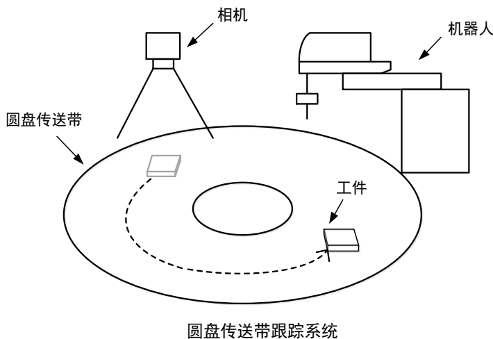
图12-10 圆盘传送带跟随系统示意
